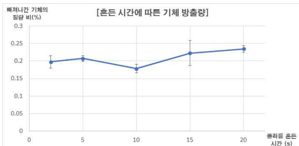
[그림 14] 콜라를 흔든 시간에 따른 기체 방출량 3회 평균 및 표준 편차
