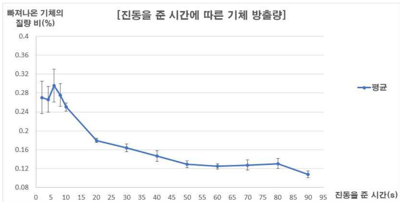
[그림 36] 콜라를 5초 흔들고 진동을 준 후 열었을 때 기체 방출량(3회 반복)
