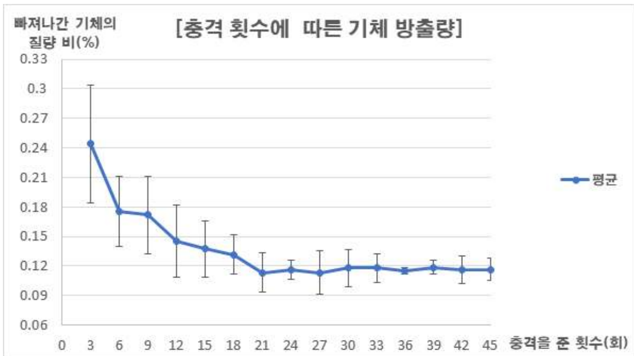
[그림 28] 콜라를 5초 흔들고 충격을 준 후 열었을 때 기체 방출량(3회 반복)
