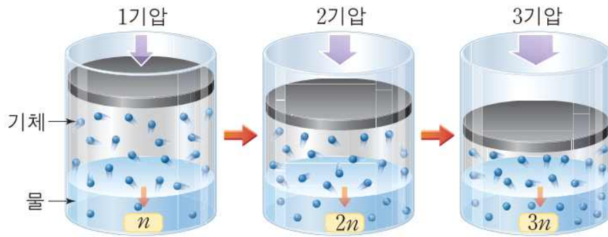
[그림 1] 압력에 따른 기체의 용해도
